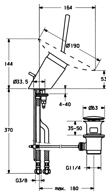
Produktzeichnung
